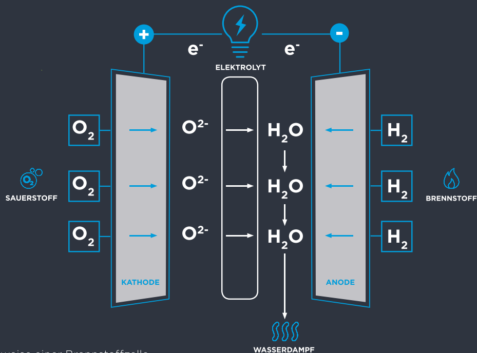
Abb. Funktionsweise einer Brennstoffzelle
